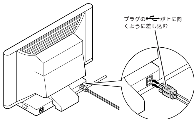
TVチューナ内蔵ワイド液晶ディスプレイ
